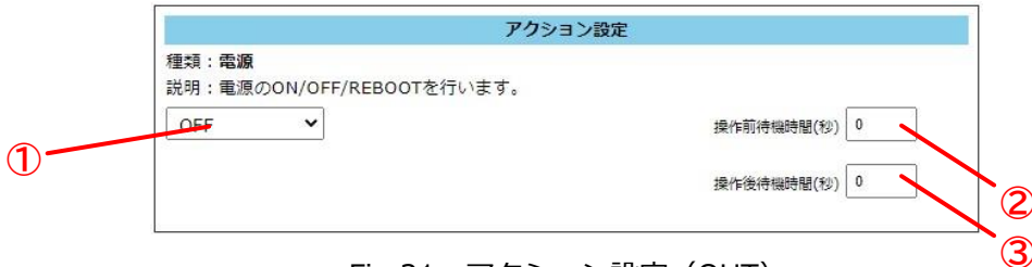
Fig.21 アクション設定 (OUT)
