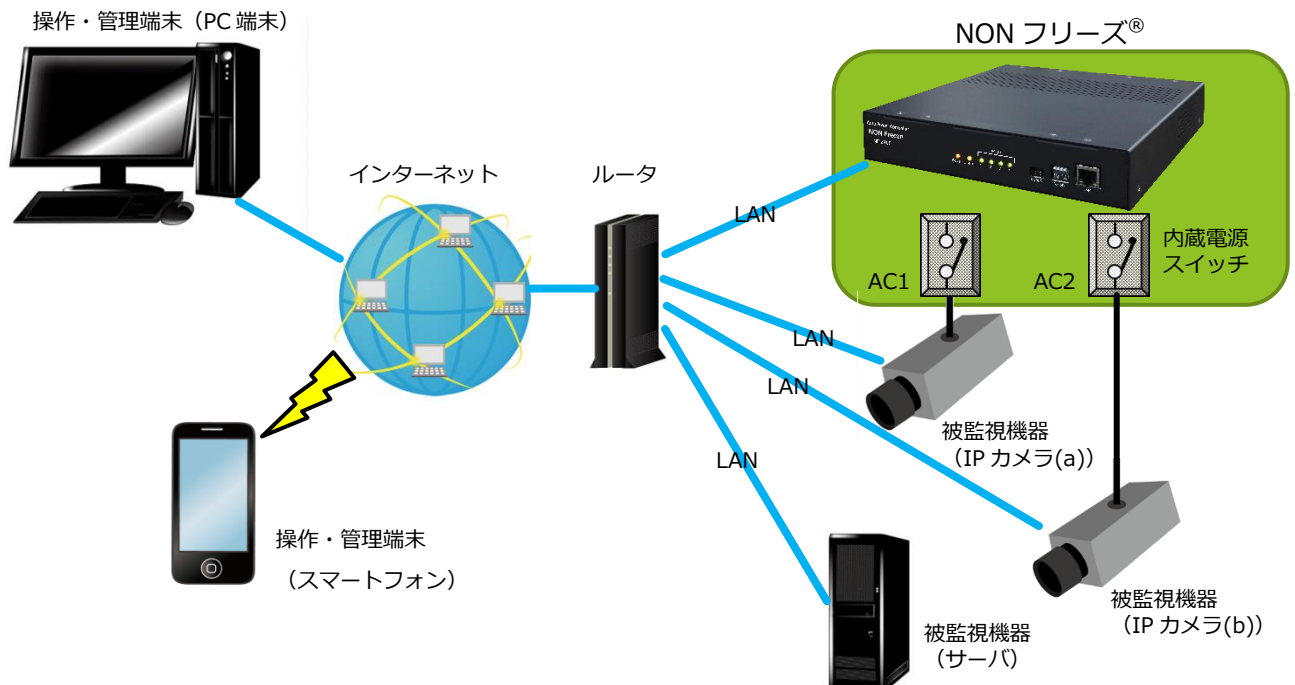
Fig.1 システム構築例
