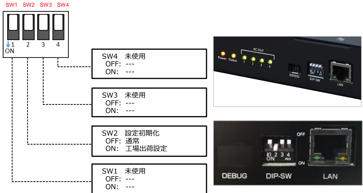
Fig.7 DIP スイッチ設定
